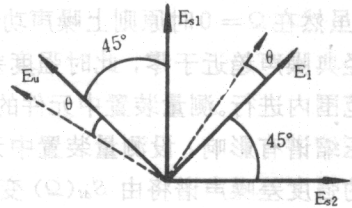
Fig. 3 The polarization orientation of E_{s1} 、 E_{s2} 、 E_1 and E_v
